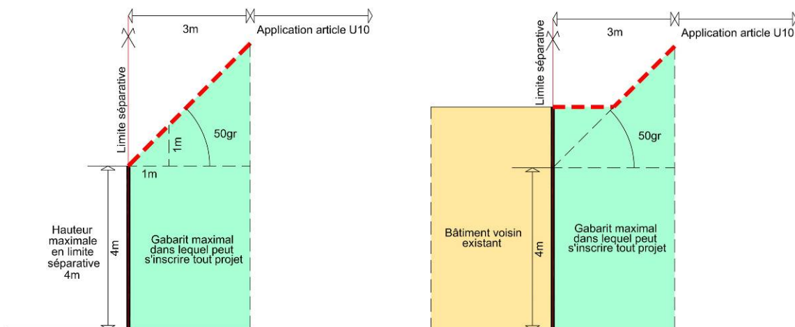
Coupe hors présence d'un bâtiment voisin Coupe en présence d'un bâtiment voisin
